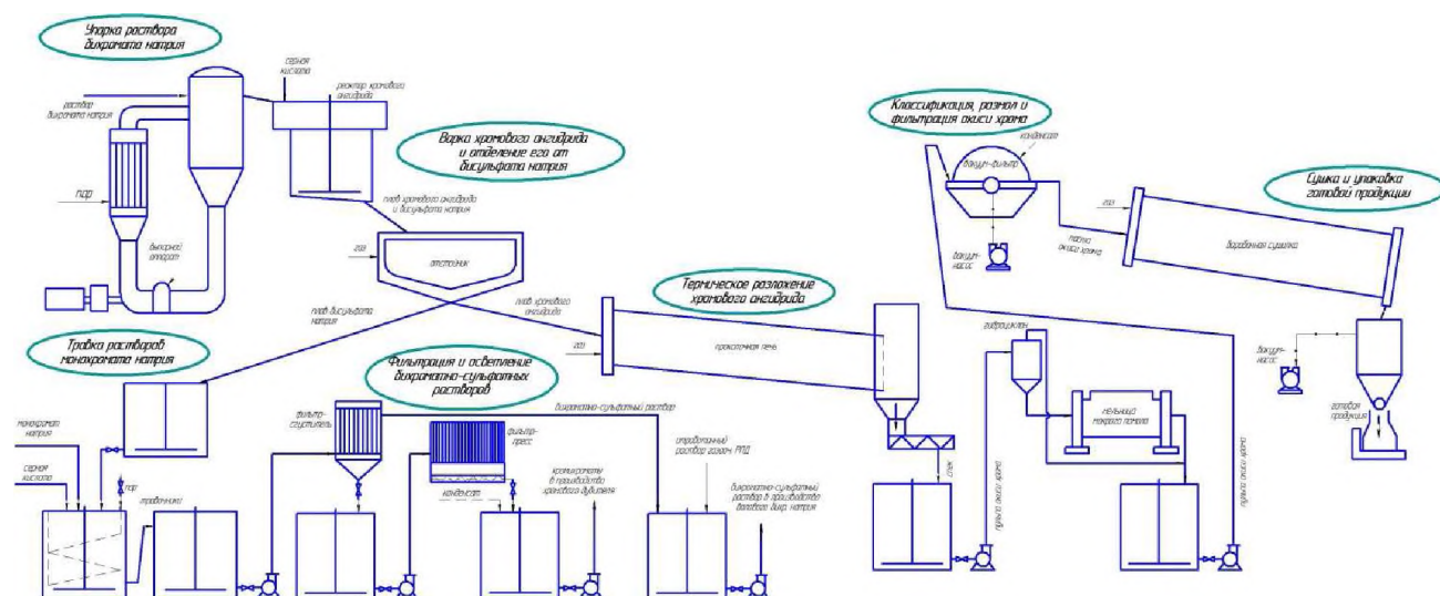
Рисунок 8.6 – Принципиальная схема производства пигментной окиси хрома
