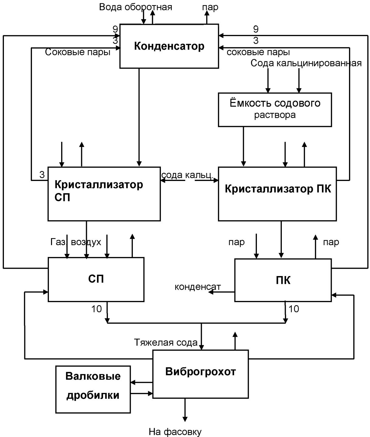
Рисунок 7.2 – Блок-схема технологического процесса производства соды кальцинированной марки А
