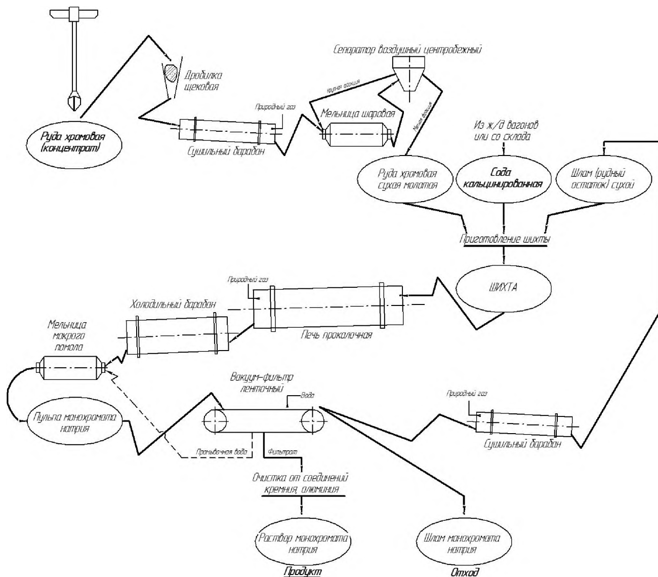
Рисунок 8.2 – Принципиальная схема получения раствора монохромата натрия (безломитовый метод)
