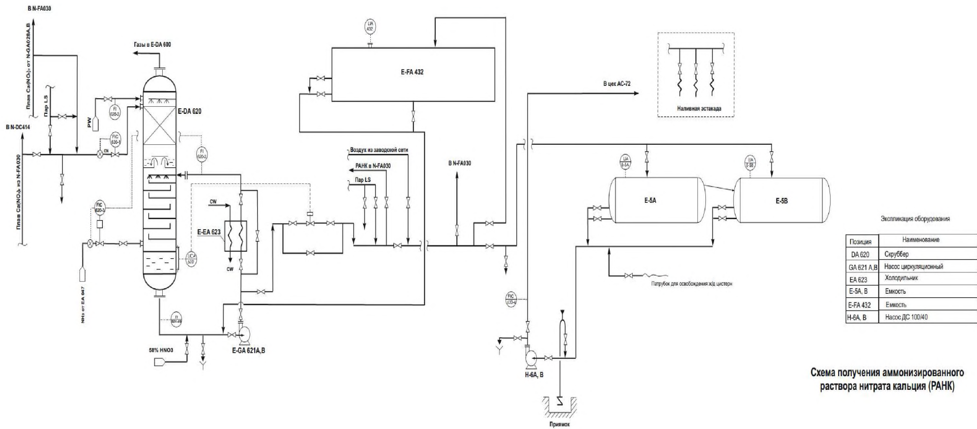
Рисунок 5.3 – Схема получения аммонизированного раствора нитрата кальция (PANК)
