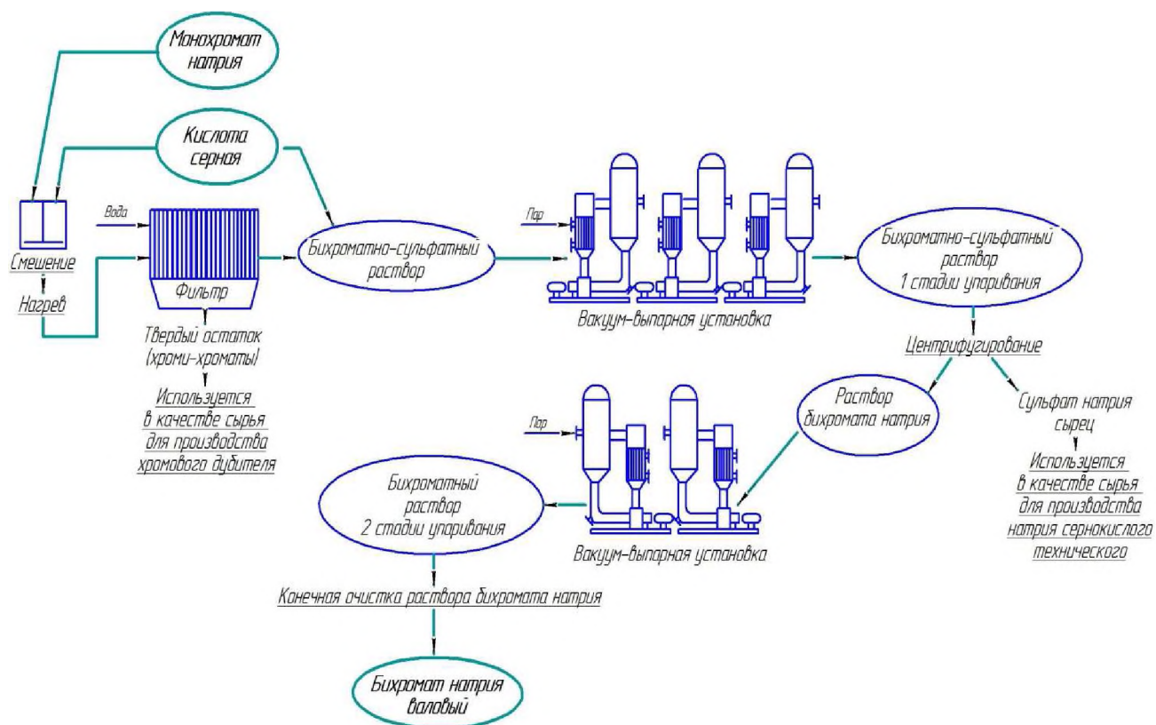
Рисунок 8.3 – Принципиальная схема производства бихромата натрия
