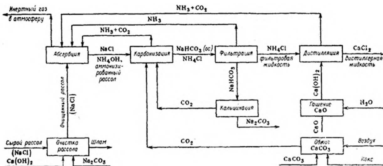
Рисунок 7.1 – Блок-схема технологического процесса производства соды
