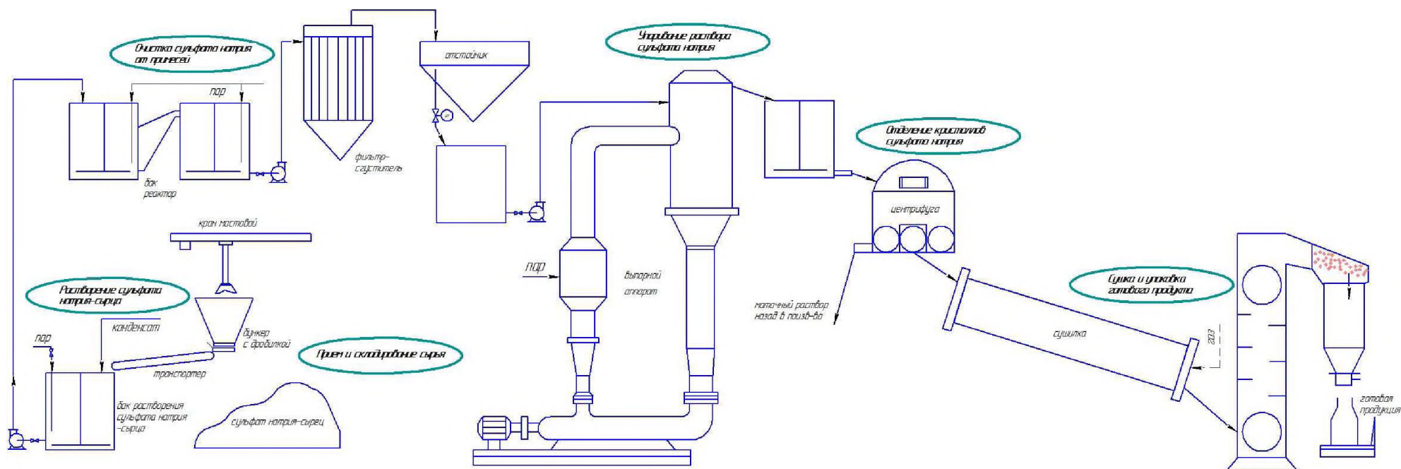
Рисунок 8.7 – Принципиальная схема производства сульфата натрия
