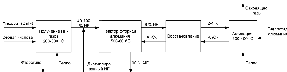
Рисунок 1.1 — Блок-схема процесса получения фторида алюминия «сухим» способом
