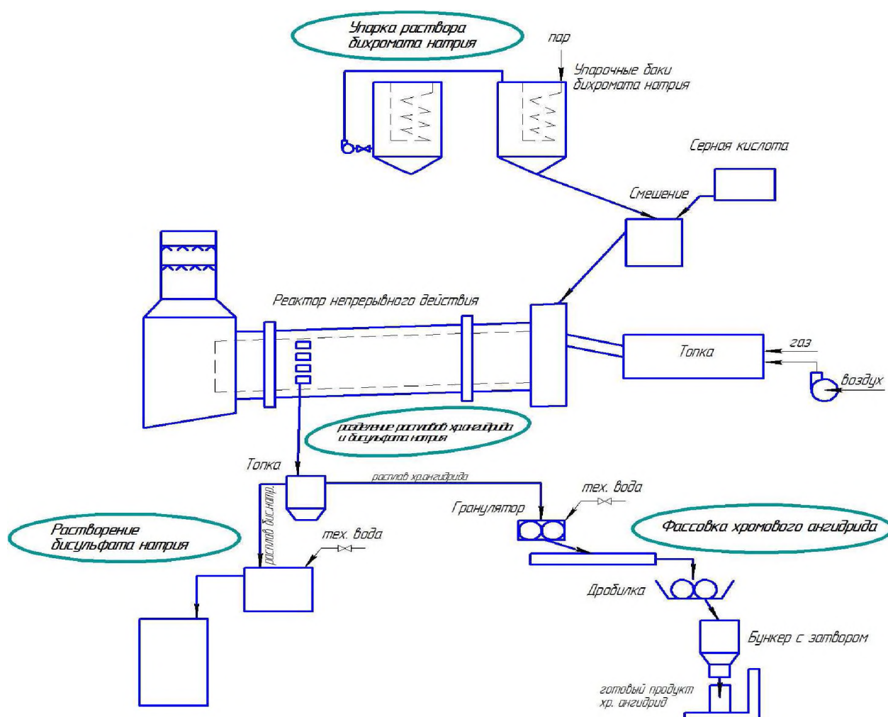
Рисунок 8.4 – Принципиальная схема производства хромового ангидрида
