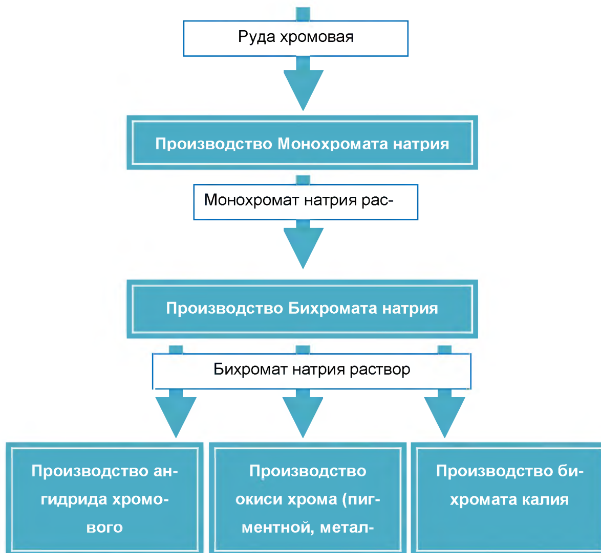
Рисунок 8.1 – Упрощенная схема связи производств основных соединений хрома между собой
