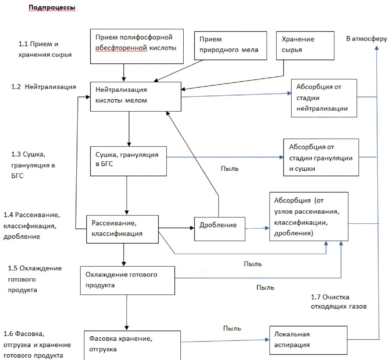
Рисунок 4.3 – Процесс производства фосфатов обезфторенных кормовых
