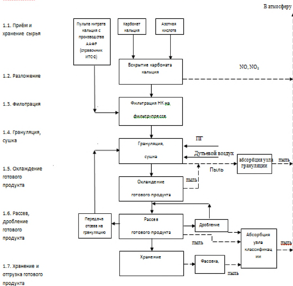
Рисунок 5.2 – Процесс производства гранулированного нитрата кальция
