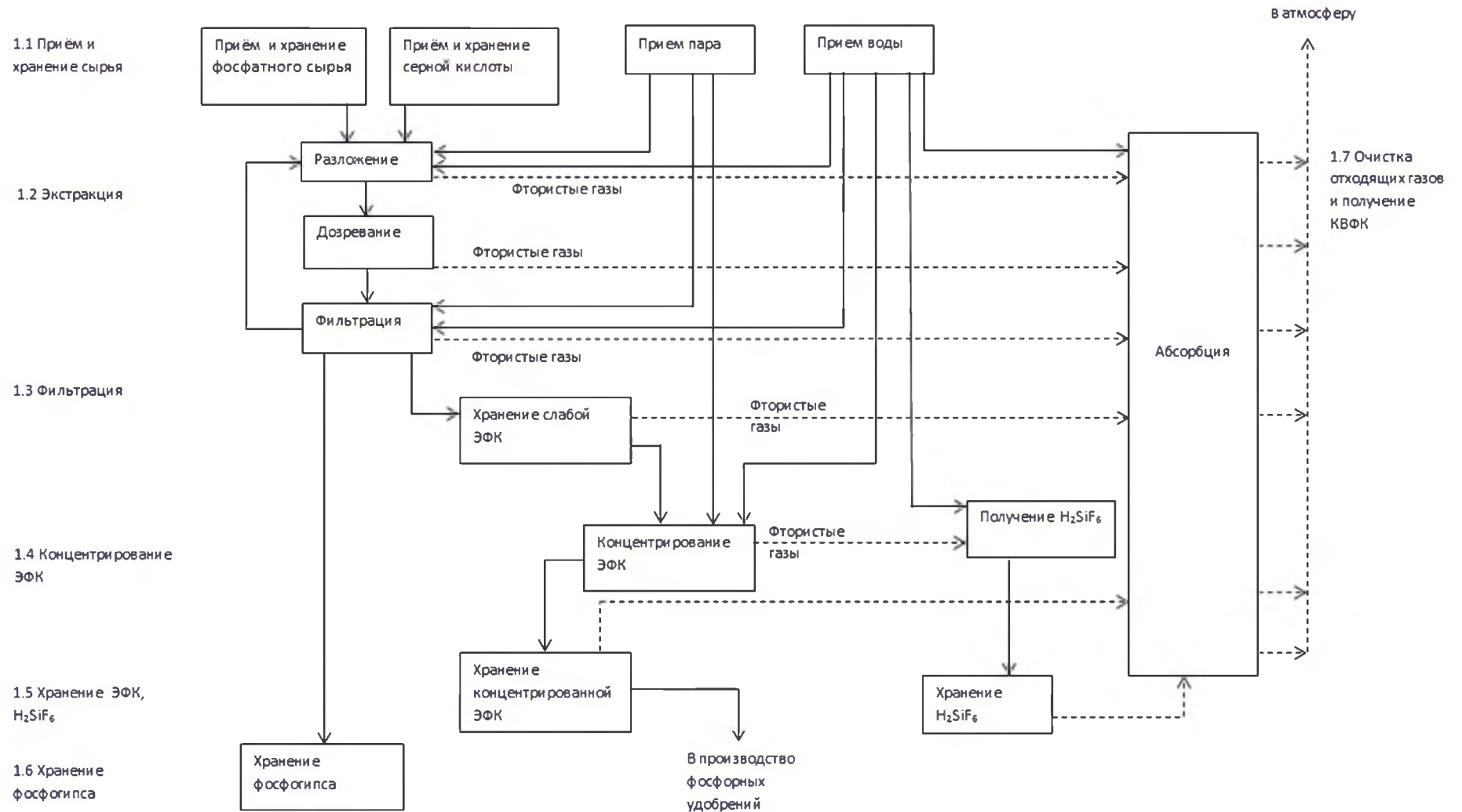
Рисунок 3.2 – Схема получения ЭФК и фосфогипса
