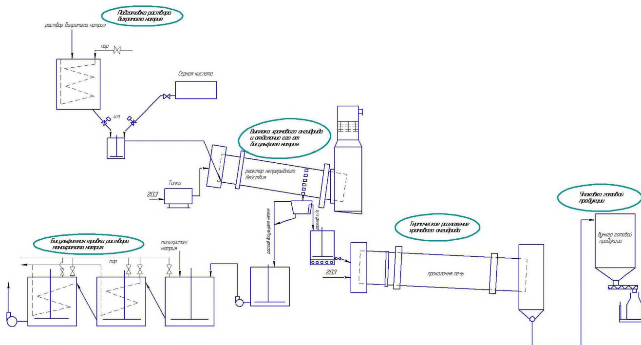
Рисунок 8.5 – Принципиальная схема производства металлургической окиси хрома
