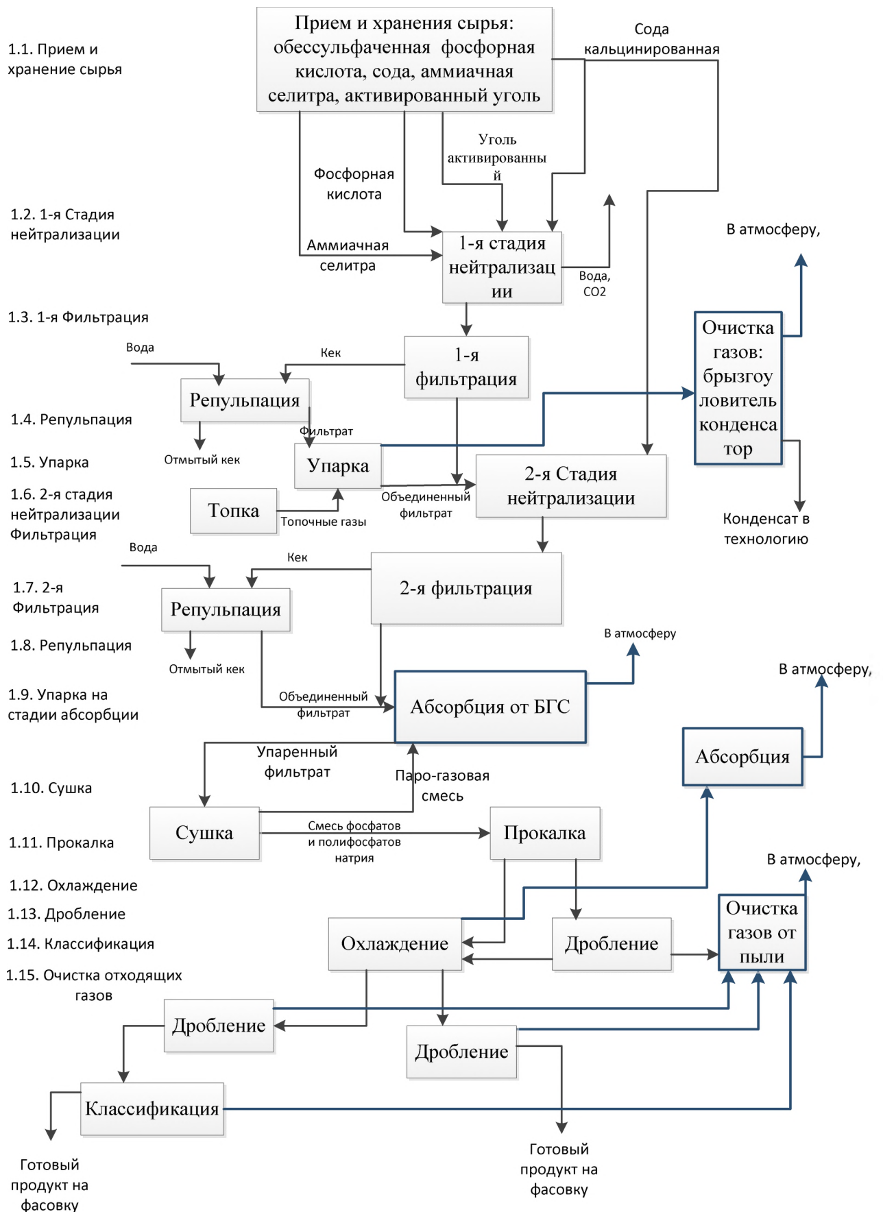
Рисунок 4.4 – Блок- схема получения ТПФН
