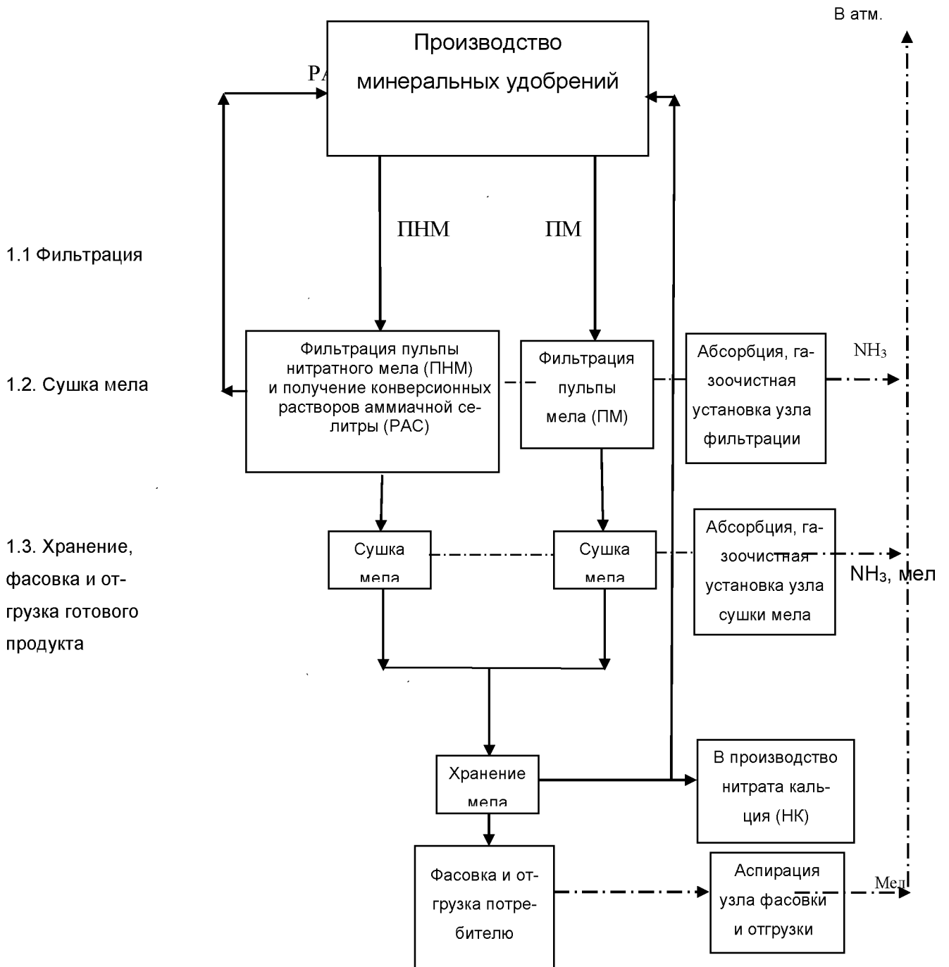
Рисунок 5.1 – Процесс производства карбоната кальция (мела)
