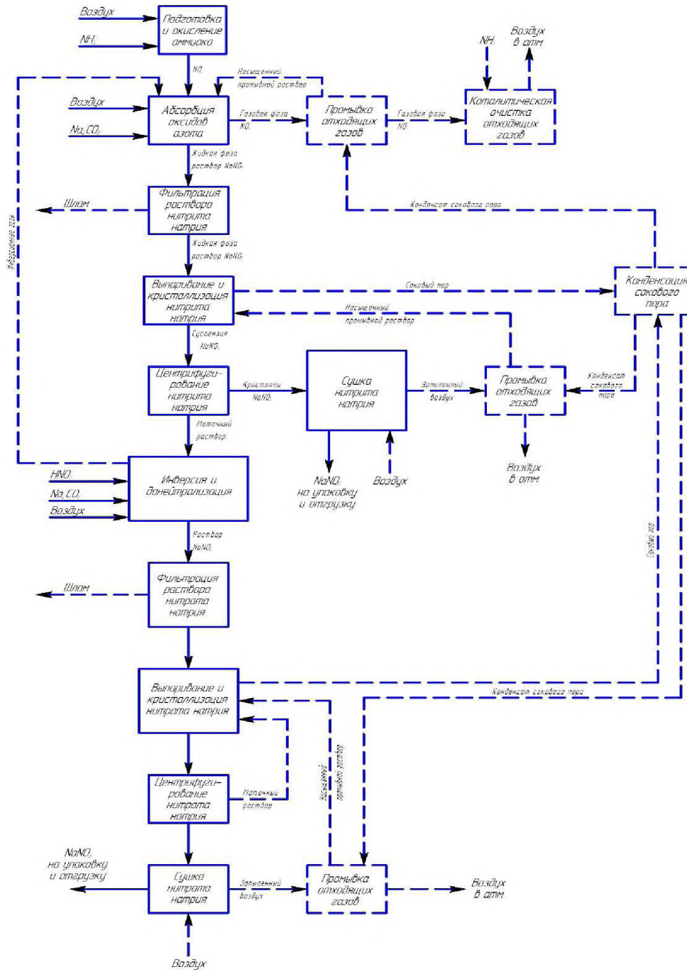
Рисунок 10.2 – Принципиальная схема производства натриевой селитры
